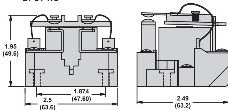
DPST-NO
